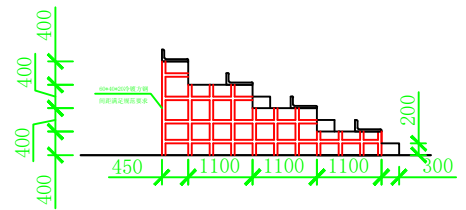
1-1剖面图
